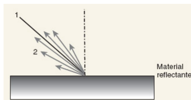
Figura 3 Retrorreflexión
